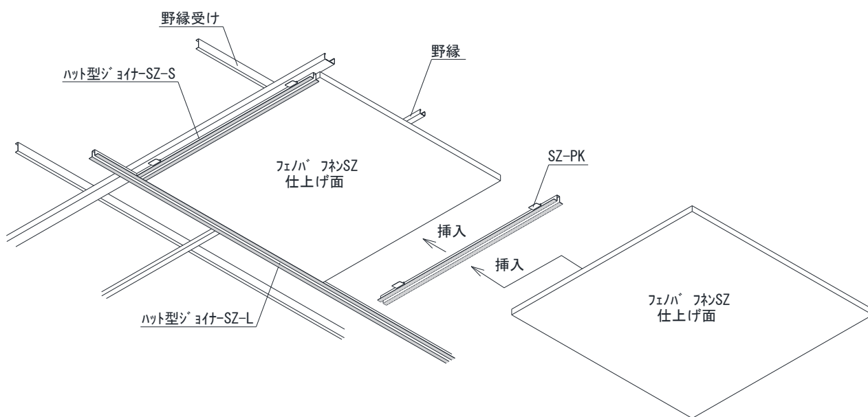
<見上げ図>
