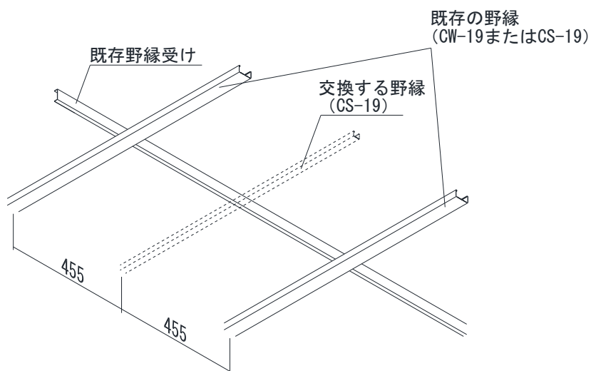
< 見上げ図 >
