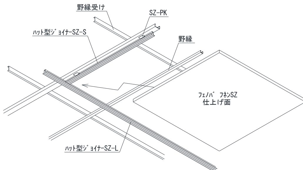
<見上げ図>
