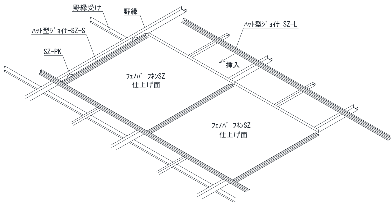
<見上げ図>
