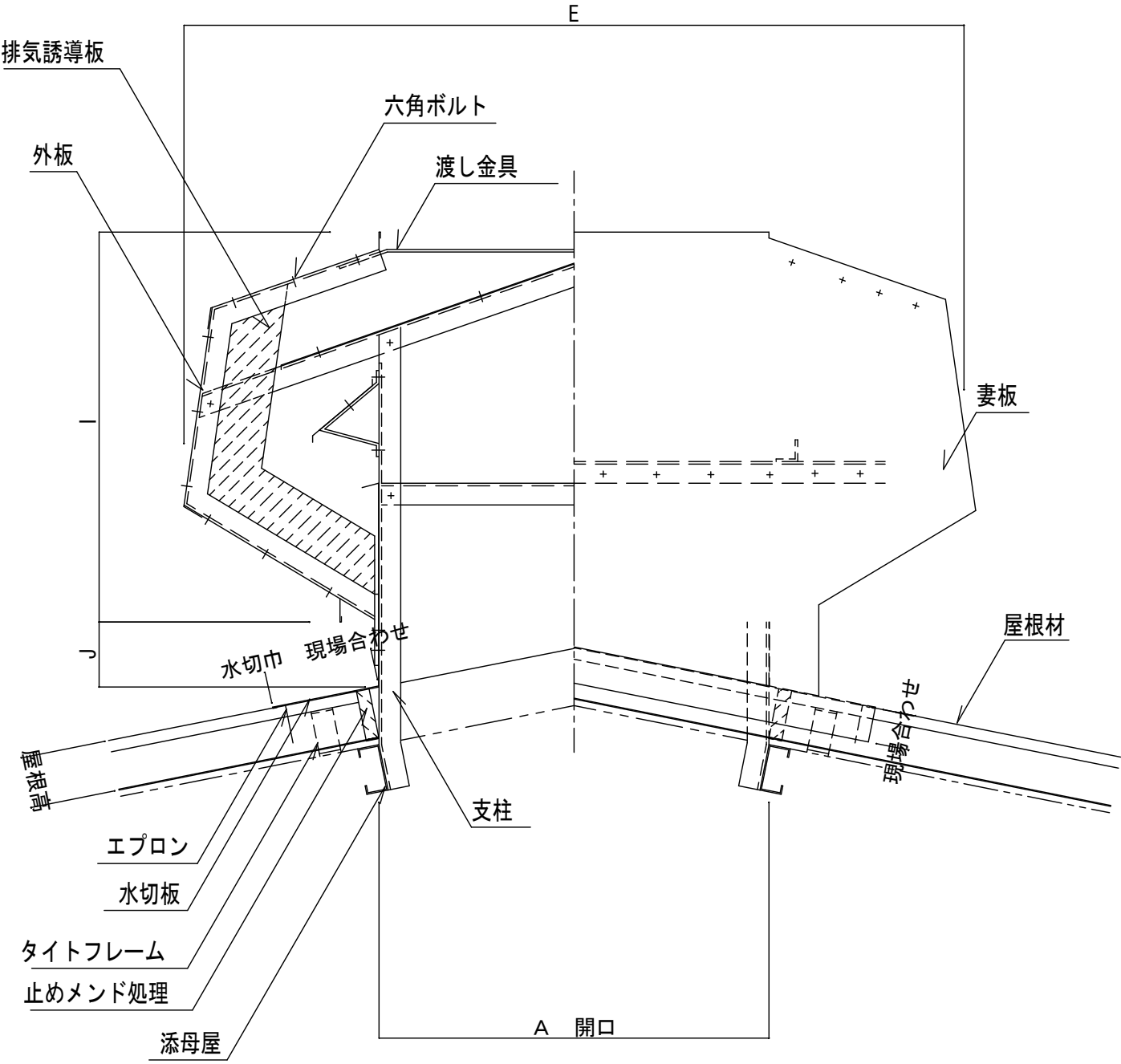
SC標準型 正面図
