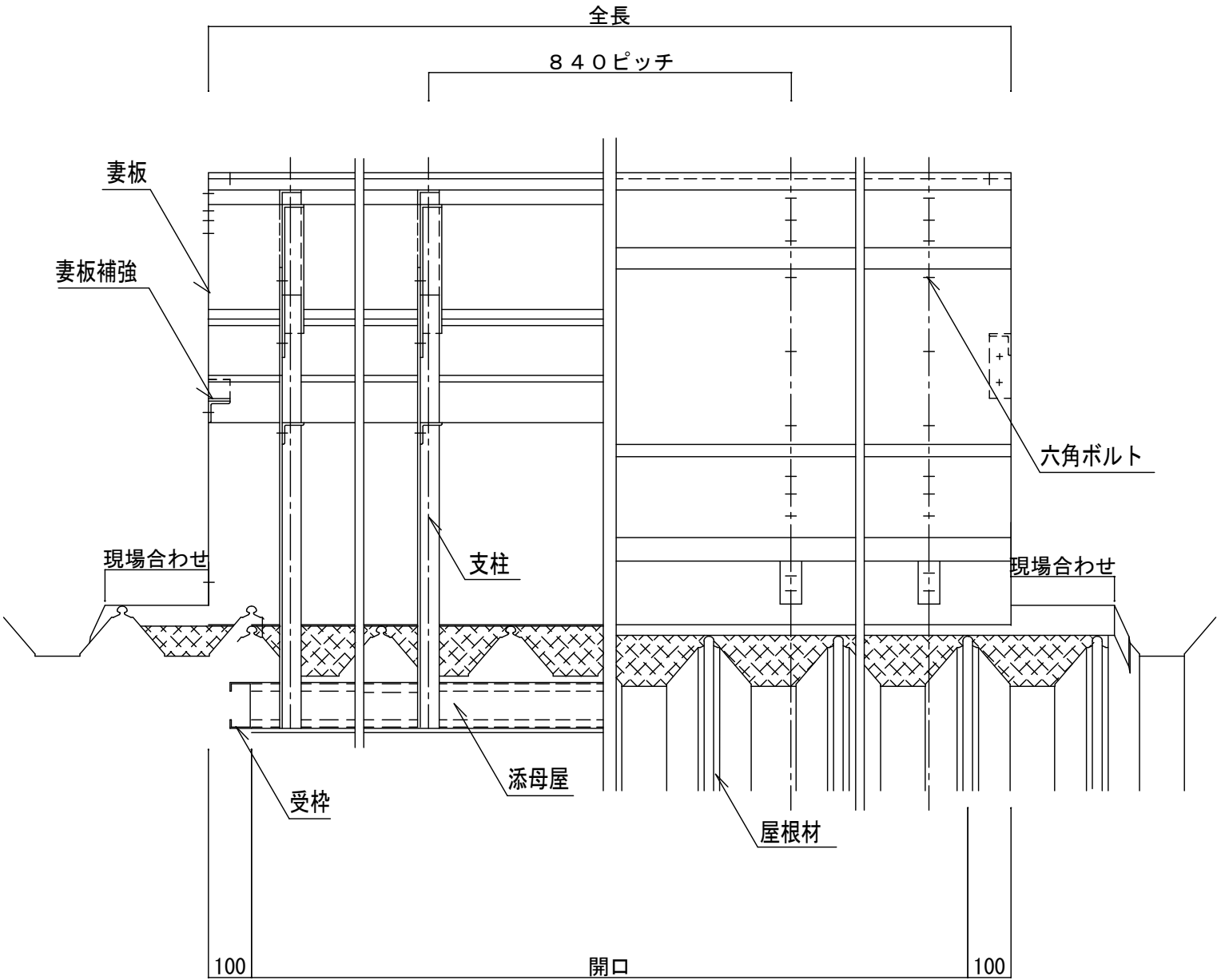
SC標準型 側面図
