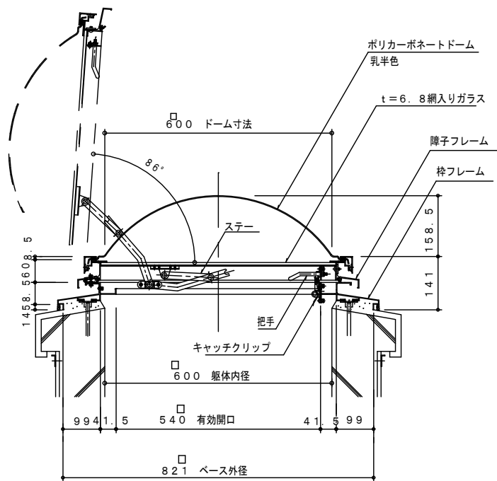
正面図 S 1 : 10
