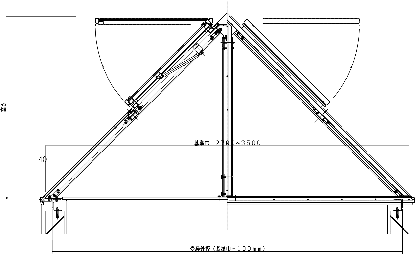
正面図
