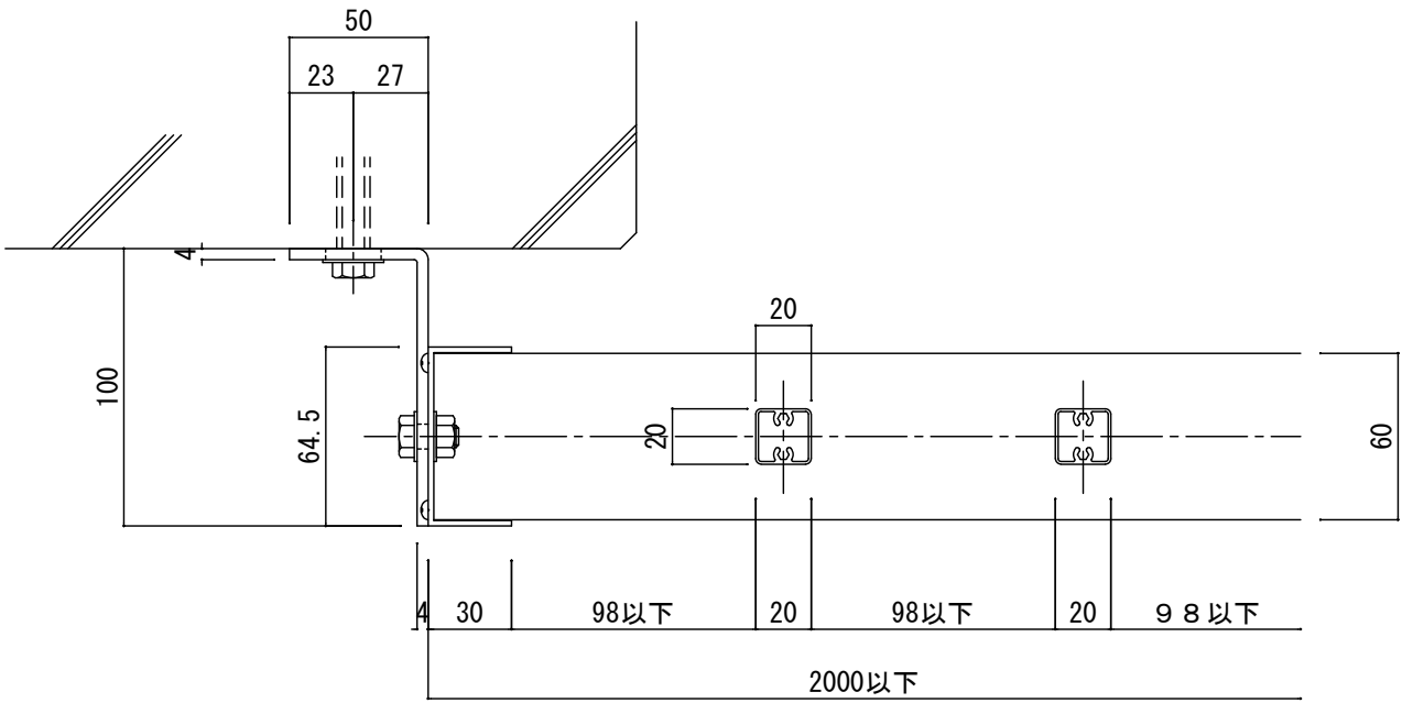
横断面図 (S : 1 / 3)
