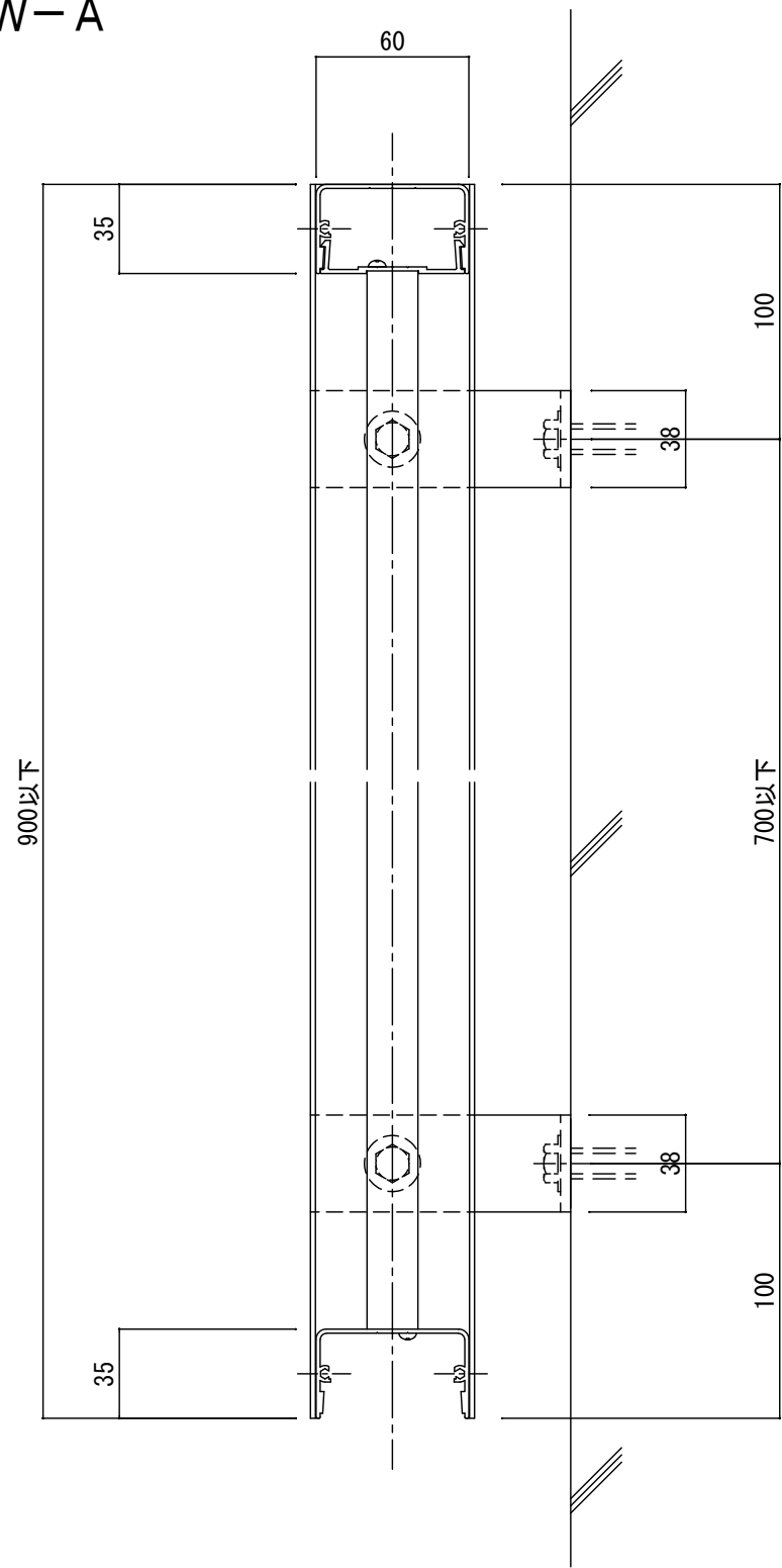
縦断面図 (S : 1 / 3)
