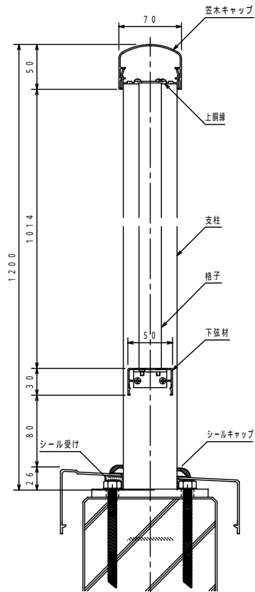
手すり断面図
