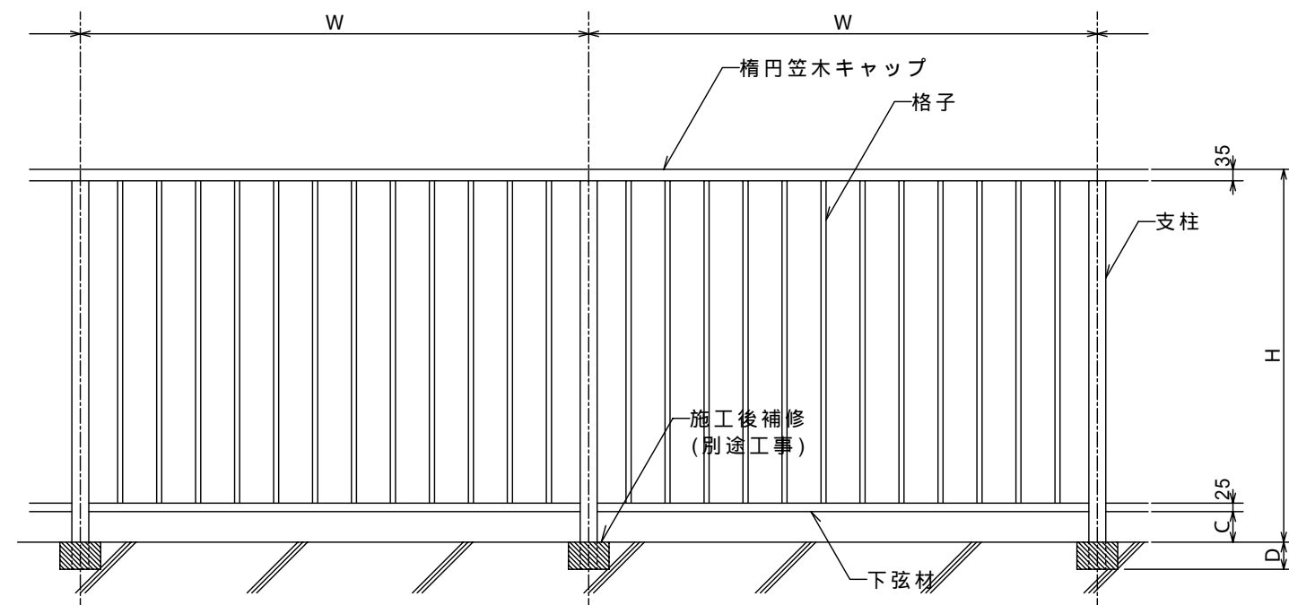
立面図 S=1/20
