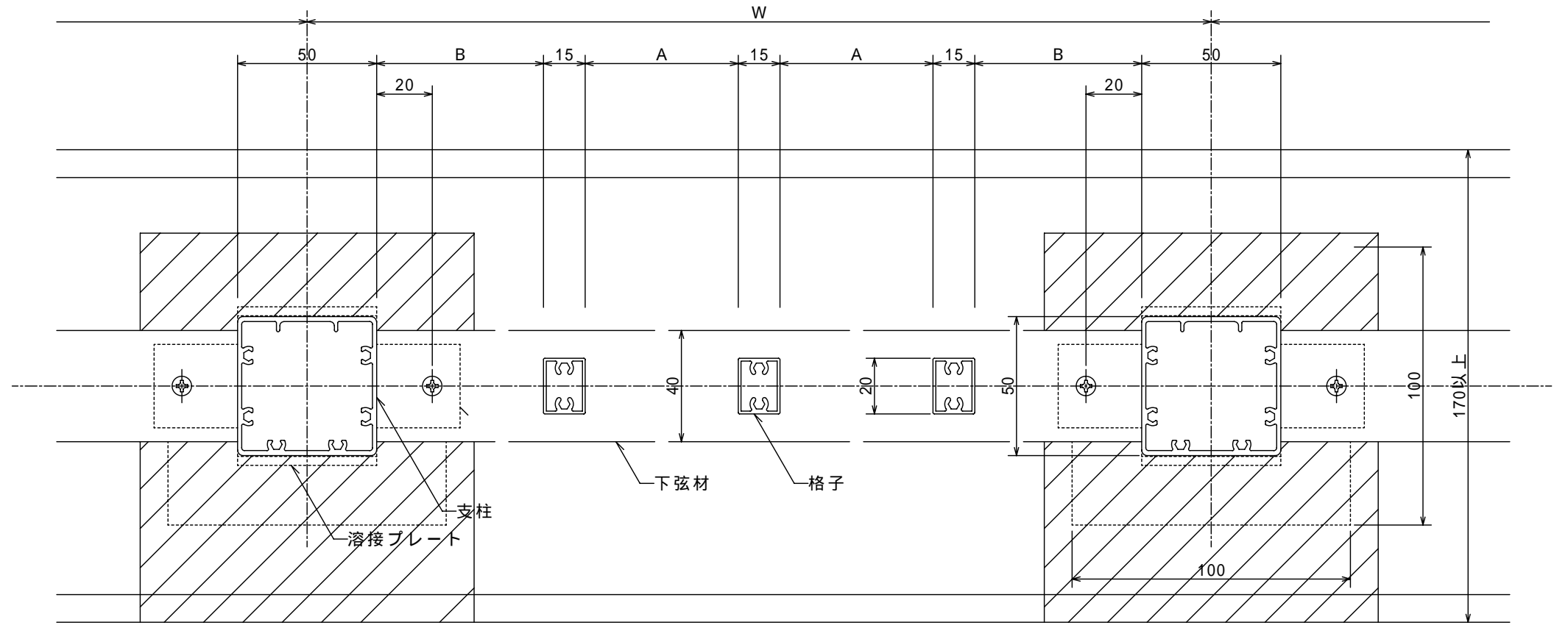
横断面図 S=1/2
