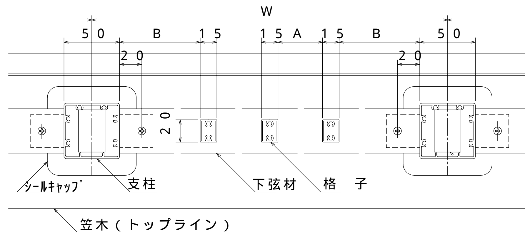
アルミ手すり付き笠木 ベースポスト方式 トップレール60A
