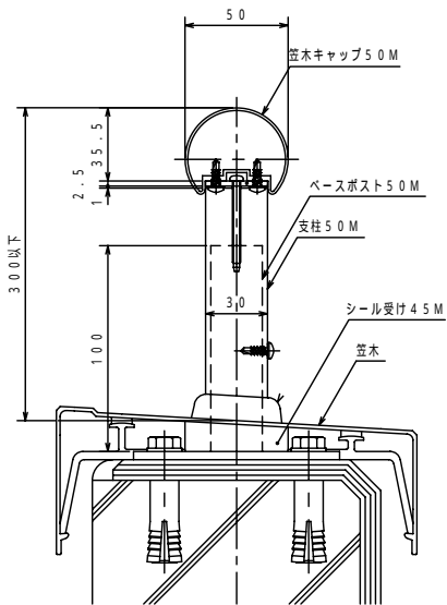
手すり断面図 (S : 1 / 2)
