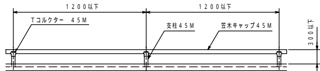
手すりユニット2スパン正面図(S:1/20)
