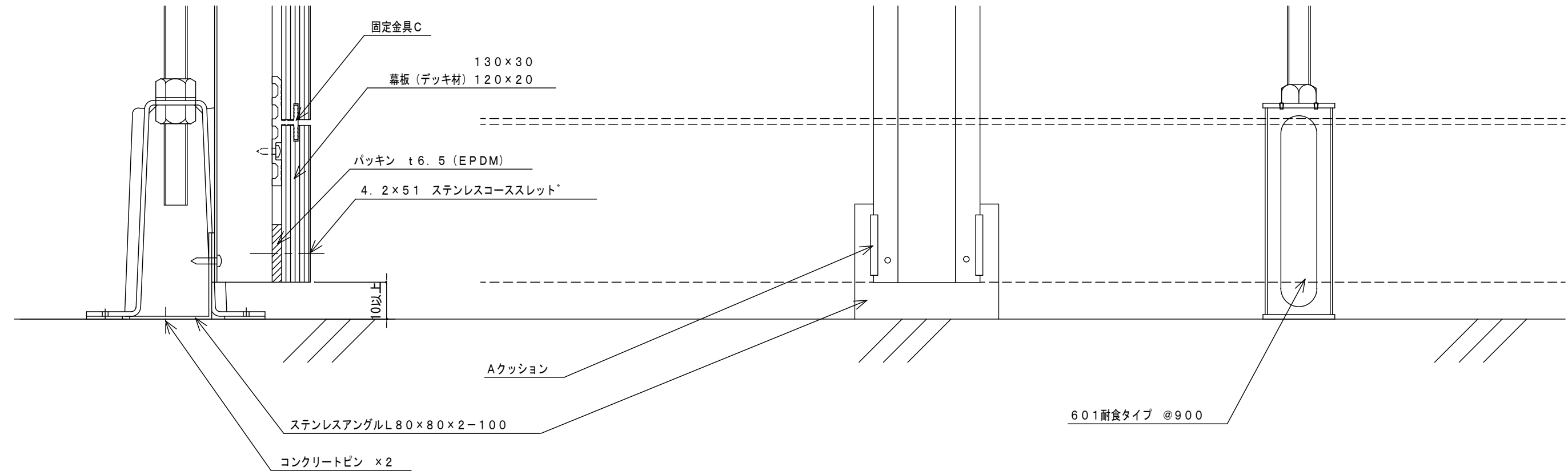
横幕板納まり図例 (デッキ床材並列方向) (縮尺: 1/3)
