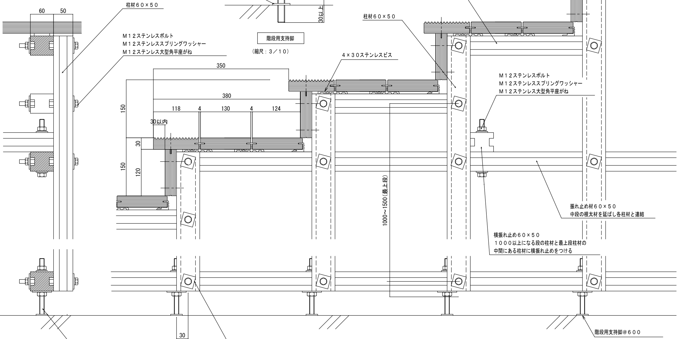
高床階段補強方法例 (縮尺: 1/5)
