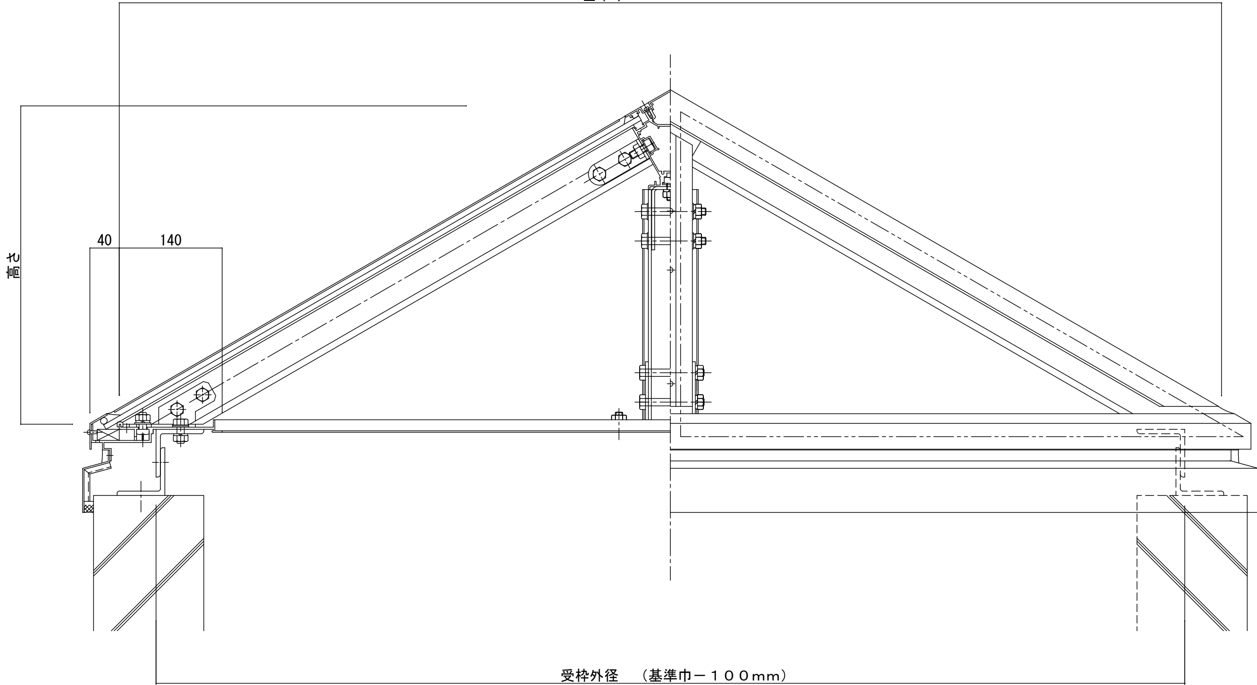
正面図
