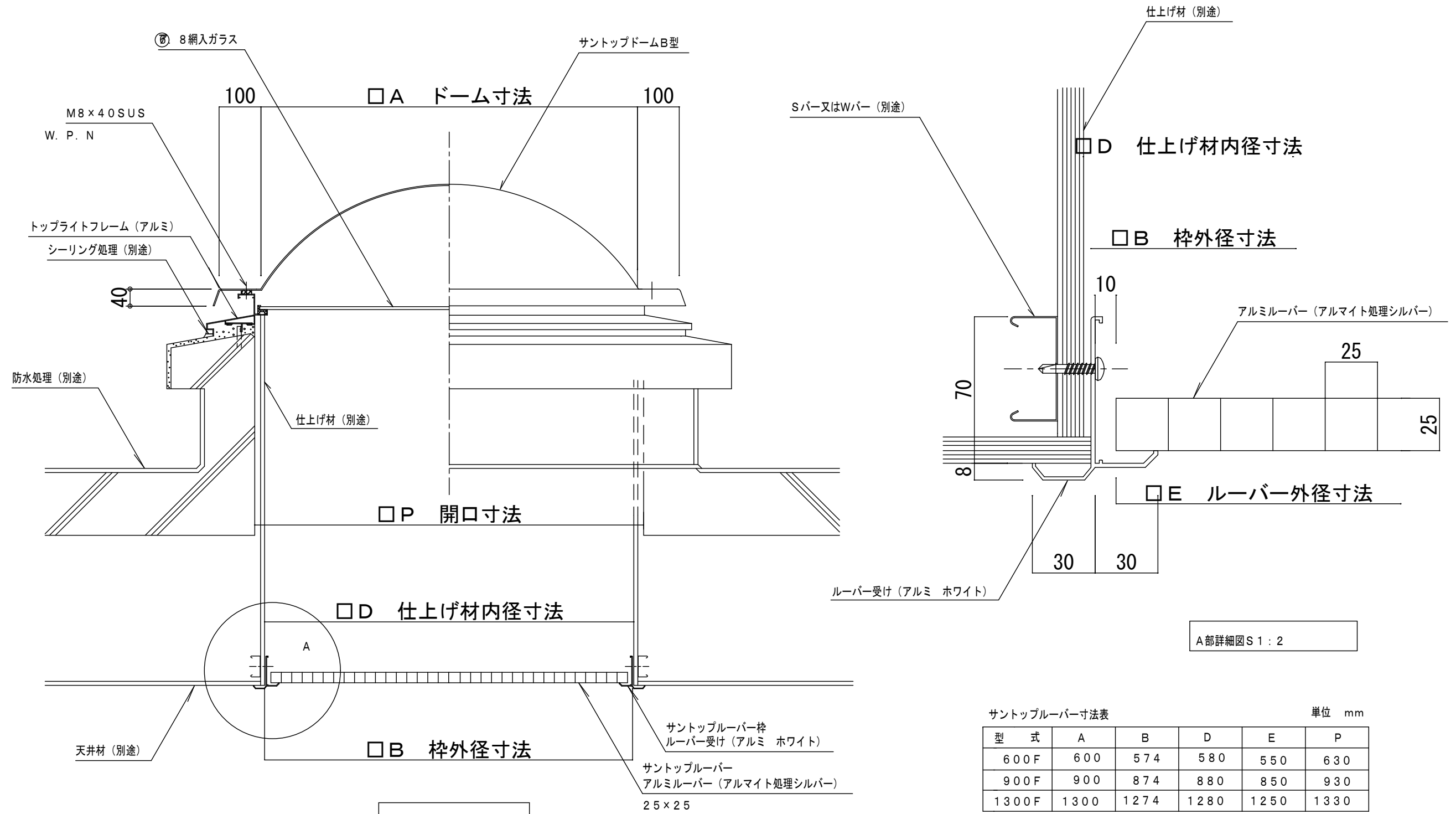
正面図S1:10
