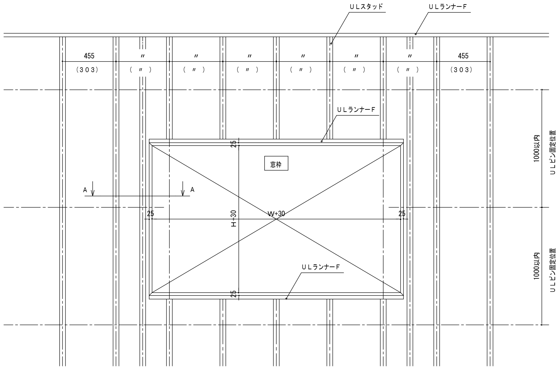
開口部納り詳細図
