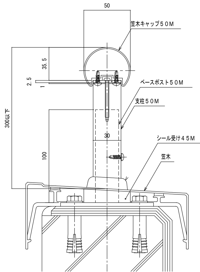
手すり断面図 (S : 1 / 2)
