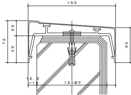
SL-150E (t=1.3) S=1/2
