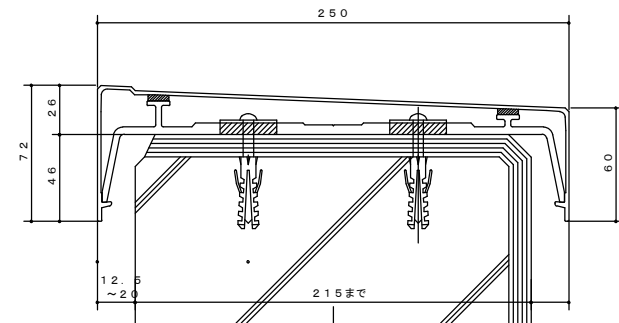
SL-250E (t=1.8) S=1/2 SL-250K (t=2.2) S=1/2
