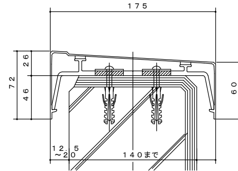
SL-175E (t=1.4) S=1/2 SL-175K (t=2.0) S=1/2
