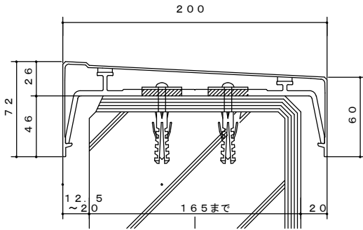
SL-200E (t=1.5) S=1/2 SL-200K (t=2.0) S=1/2
