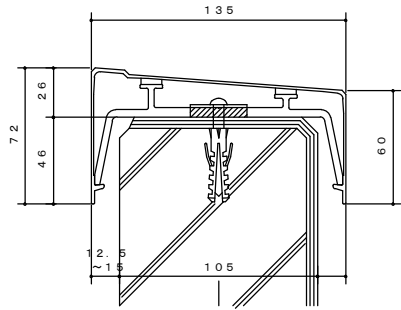
SL-135E (t=1.3) S=1/2
