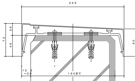
SL-225E (t=1.6) S=1/2 SL-225K (t=2.0) S=1/2
