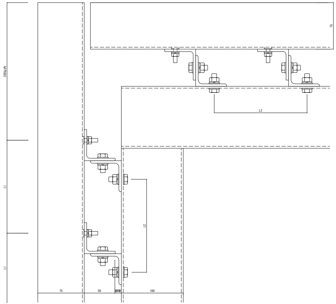
SKカクパネル KP-30横ばり
