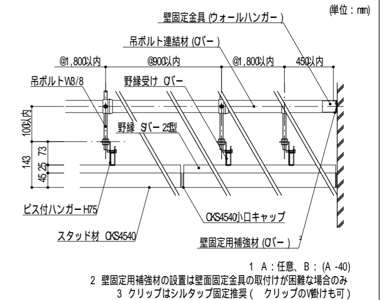
CKS4540 クリップ固定納まり図 (S:1/12)
