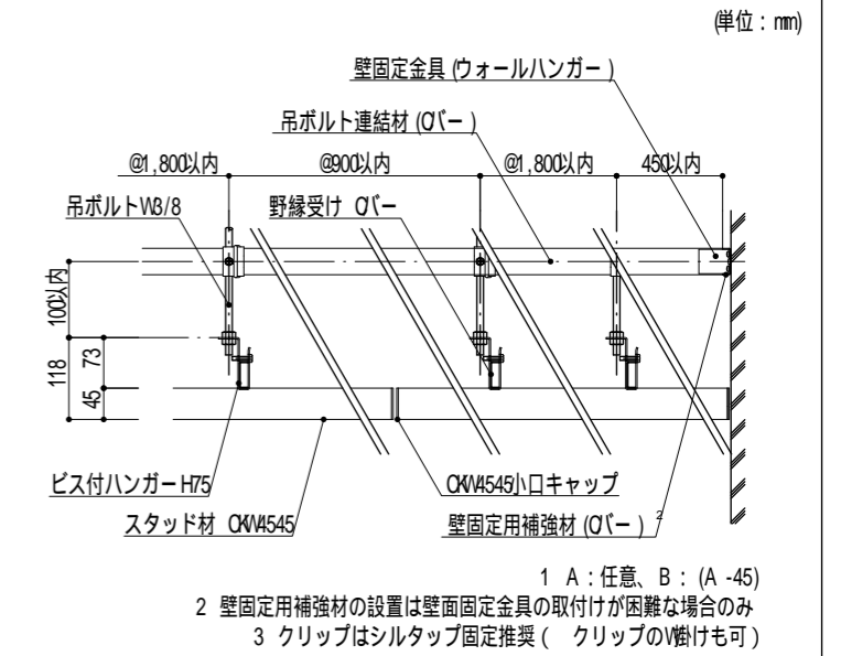
CKW4545 クリップ固定納まり図 (S:1/12)
