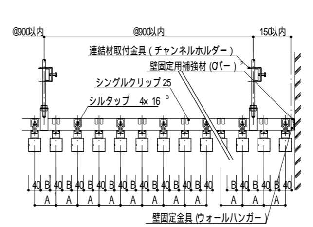
CKS4540 クリップ固定納まり図 (S:1/12)
