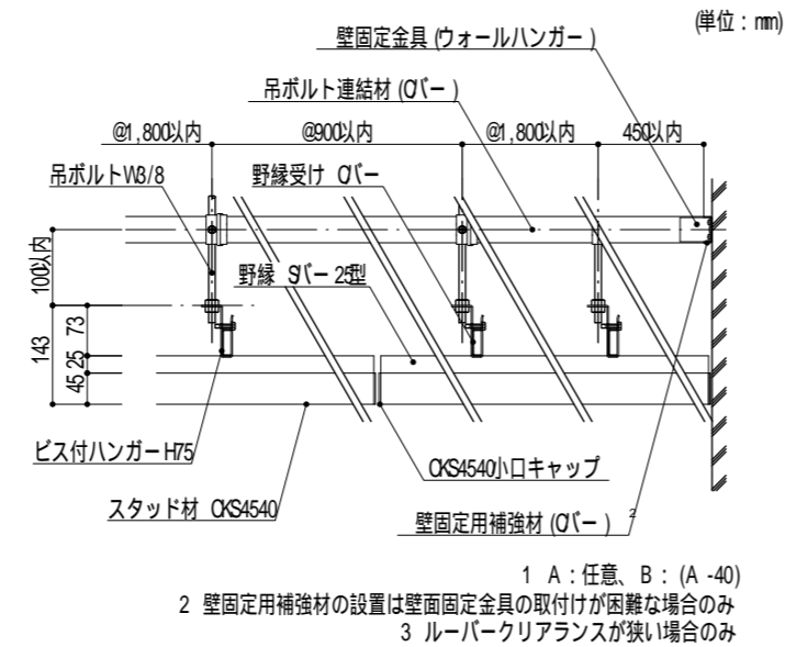
CKS4540 耐風圧クリップ固定納まり図 (S:1/12)
