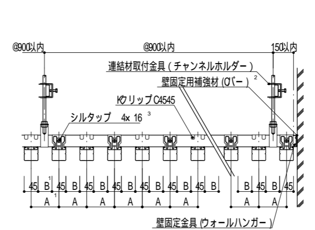
CKW4545 クリップ固定納まり図 (S:1/12)
