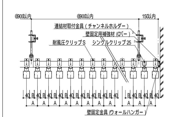
CKS4540 耐風圧クリップ固定納まり図 (S:1/12)
