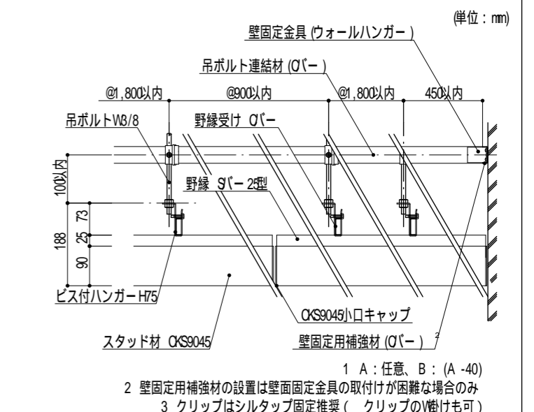
CKS9045 クリップ固定納まり図 (S:1/12)
