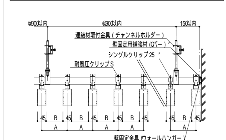
CKS9045 耐風圧クリップ固定納まり図 (S:1/12)
