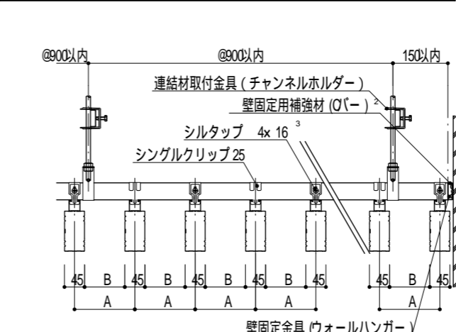
CKS9045 クリップ固定納まり図 (S:1/12)
