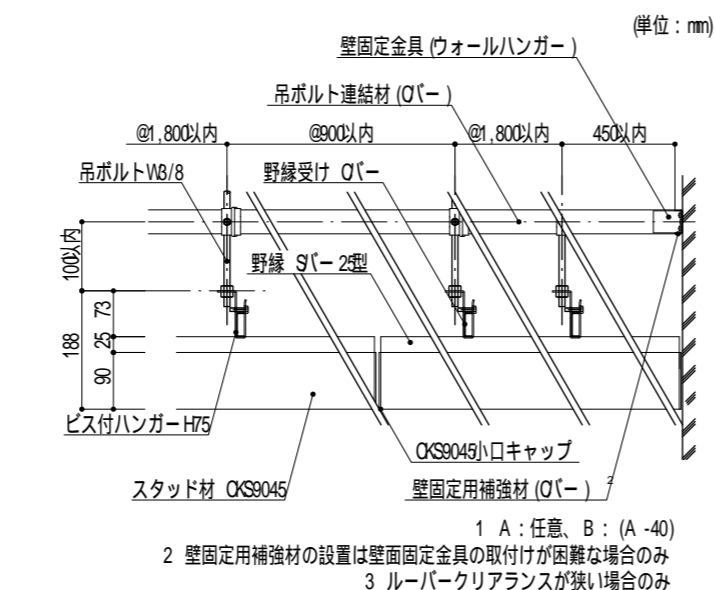
CKS9045 耐風圧クリップ固定納まり図 (S:1/12)
