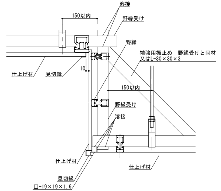
下がり壁と野縁が平行の場合
