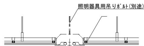
A-A' 野縁受け方向
