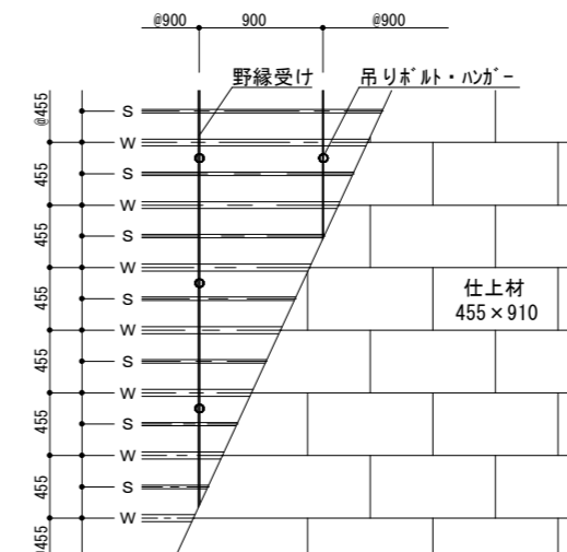
ボート直貼用下地② (W-S-W)
