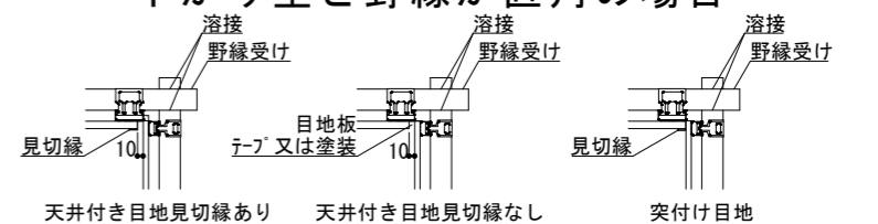
下がり壁と野縁が直角の場合
