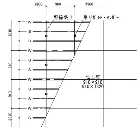
ボート直貼用下地① (W-S-S-W)
