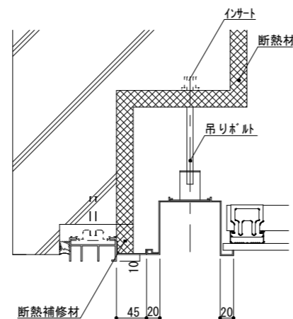
アルミニウム製埋込みタイプ
