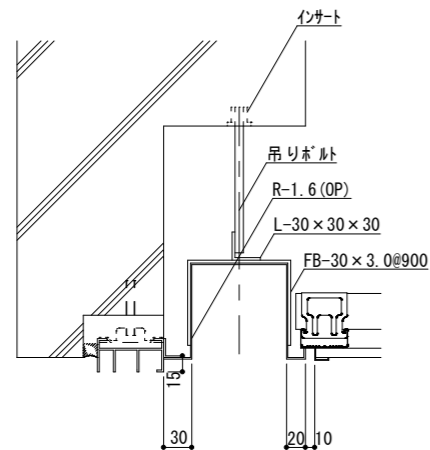
鋼製埋込みタイプ
