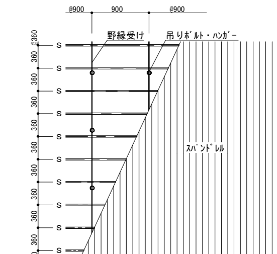
スパンドレル直貼用下地 (S-S-S-S-S-S)
