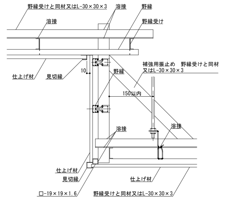
下がり壁と野縁が直角の場合
