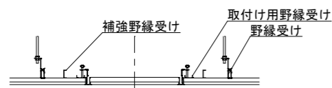
B-B' 野縁受け直交方向
