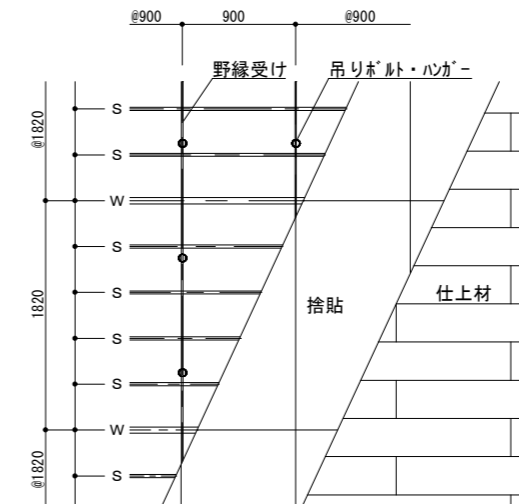
ボート & 捨貼用下地 (W-S-S-S-S-W)
