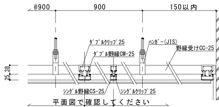
(野縁受け方向)
