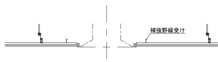
B-B' 野縁受け直交方向
