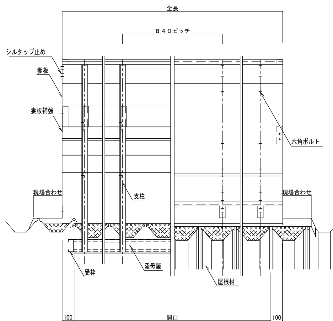
側面図
