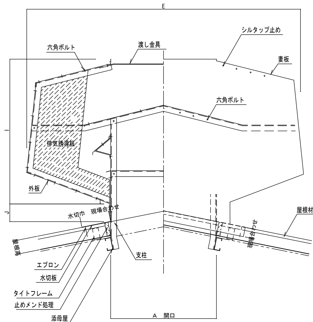
正面図
