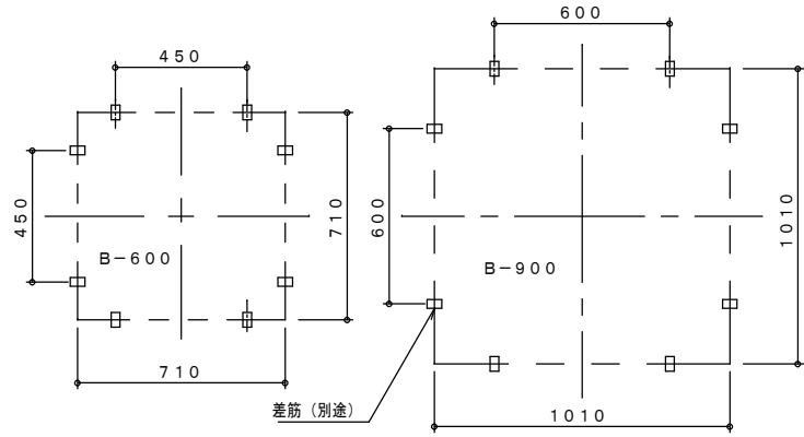
アンカー位置図 S1:20
