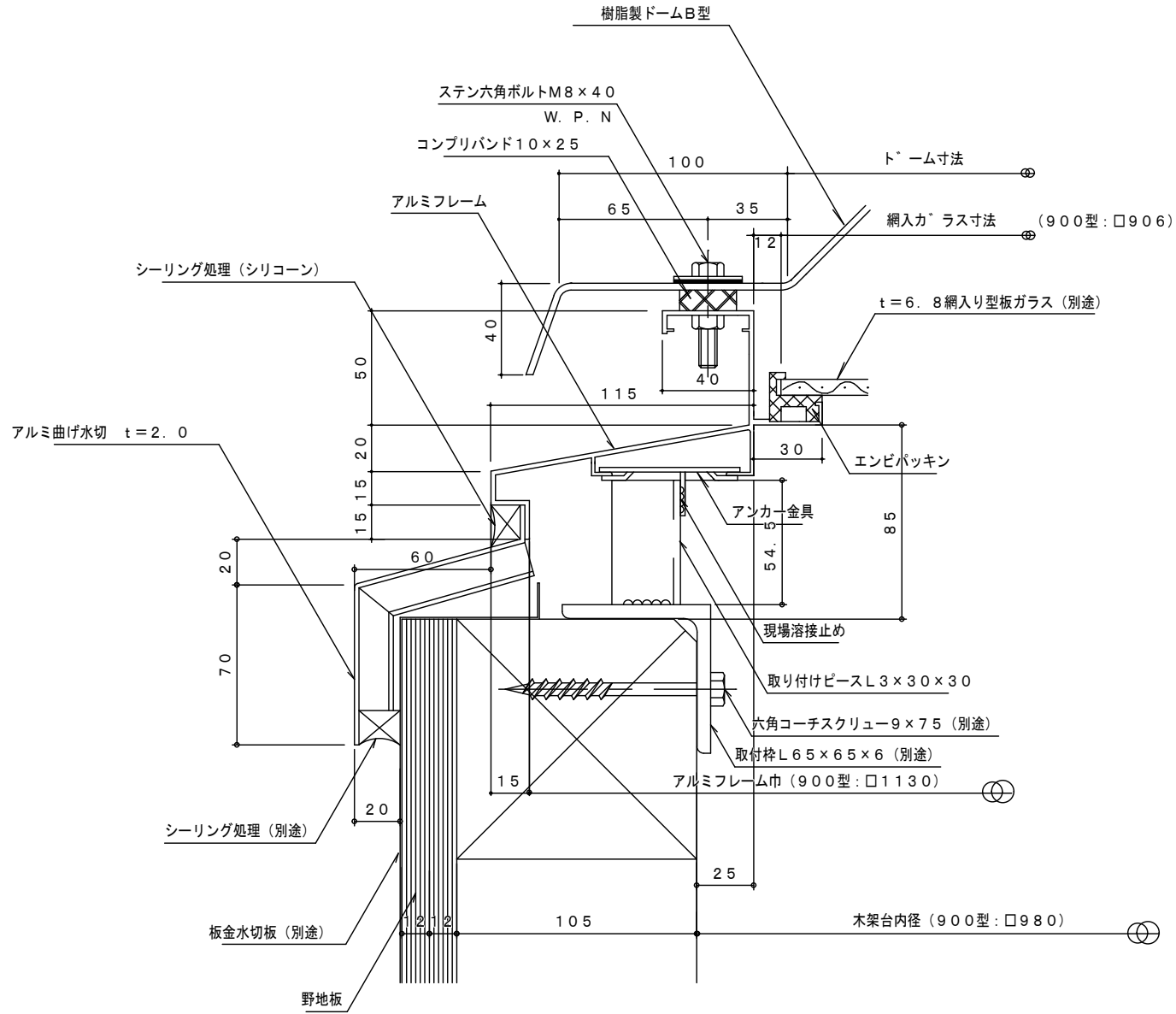
断面詳細図 S1:2
