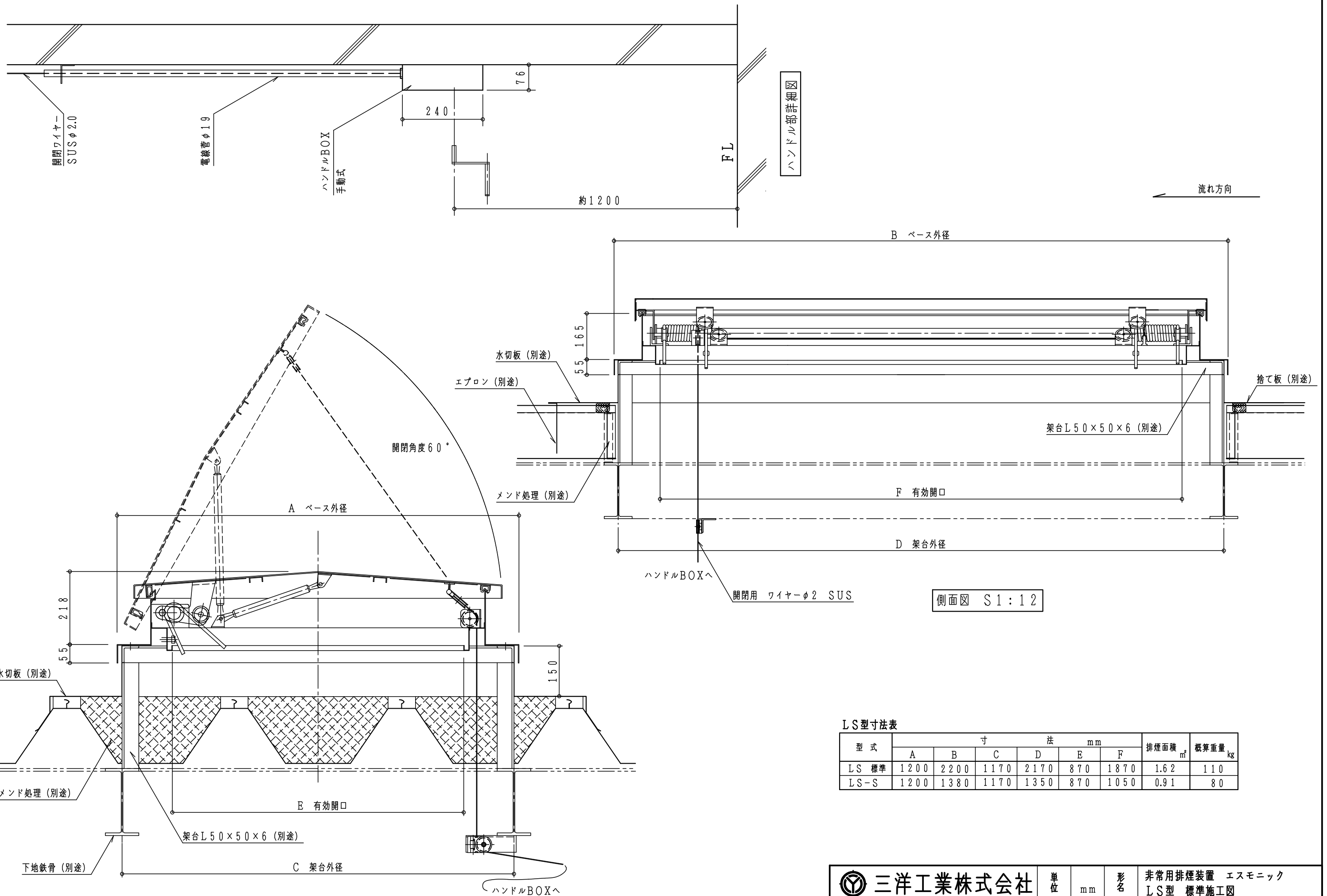
正面図 S1:10
