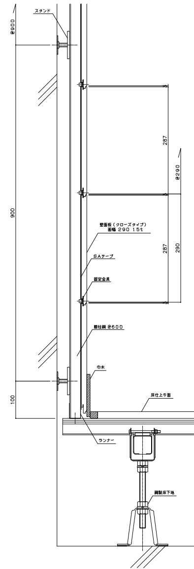
■ 緩衝内壁システム【カベックス：クローズタイプ】
