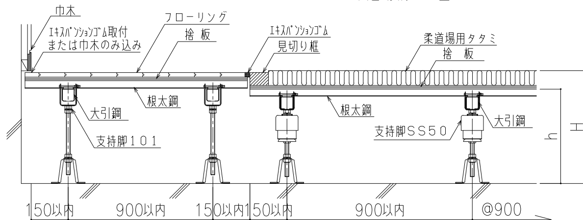
■柔道場納まり図
