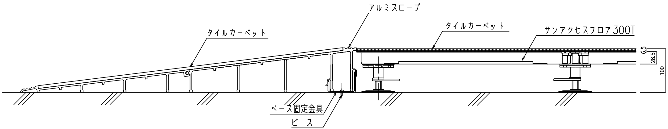
【アルミスロープ部納まり図（サンアクセスフロア 300T：モルタル充填タイプ）】
