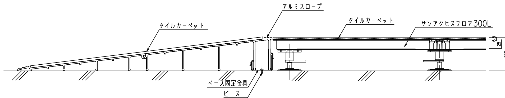
【アルミスロープ部納まり図（サンアクセスフロア 300L：中空タイプ）】
