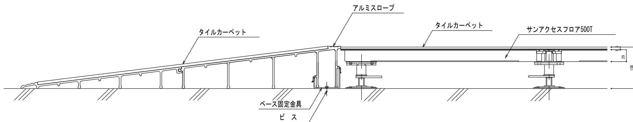
【アルミスロープ部納まり図（サンアクセスフロア 500T：モルタル充填タイプ）】
