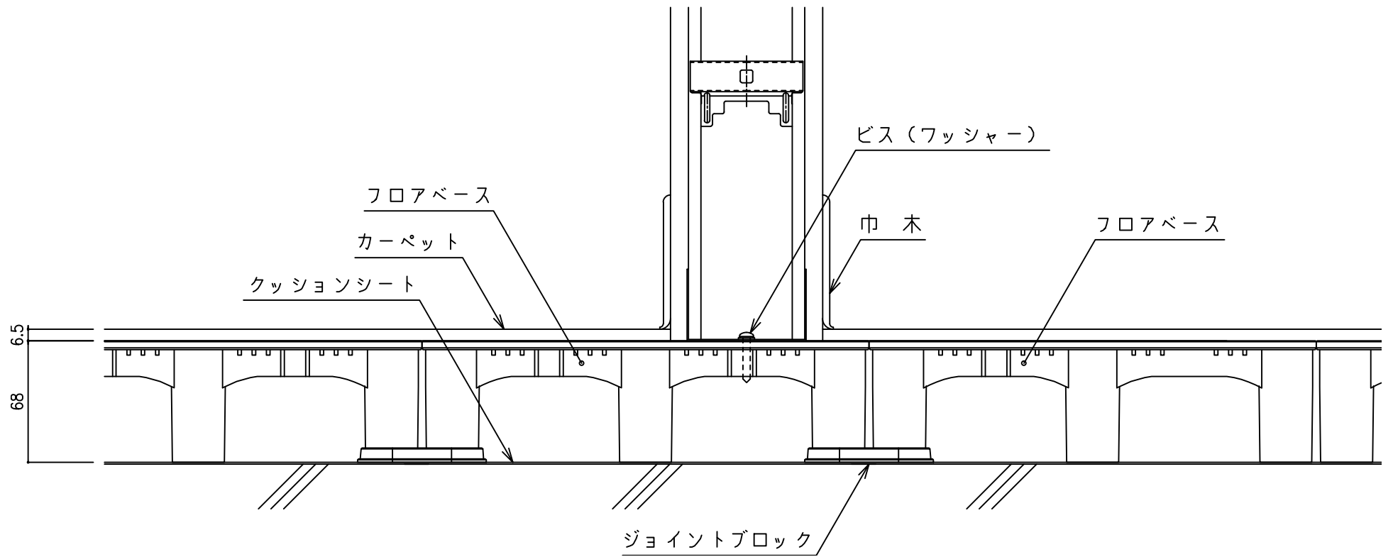
【間仕切取付け参考納まり図（フロアベースST-3000N・2000N）】
