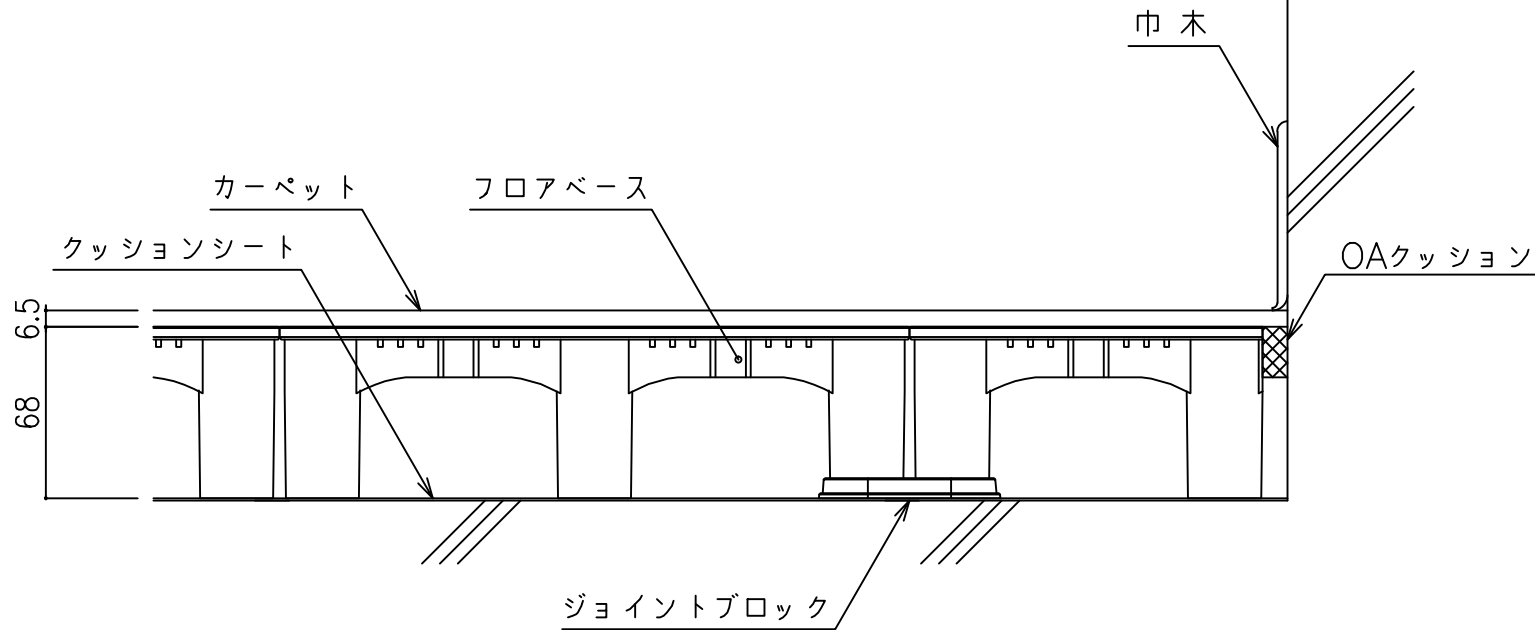
【貼り仕舞い参考納まり図（フロアベースST-3000N・2000N）】
