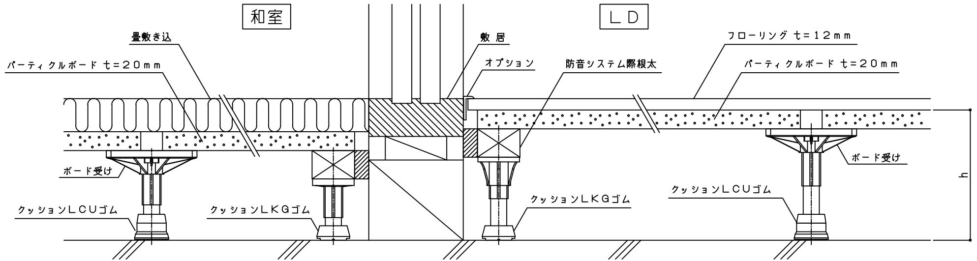
【ホームベース LCU：敷居廻り詳細図】
