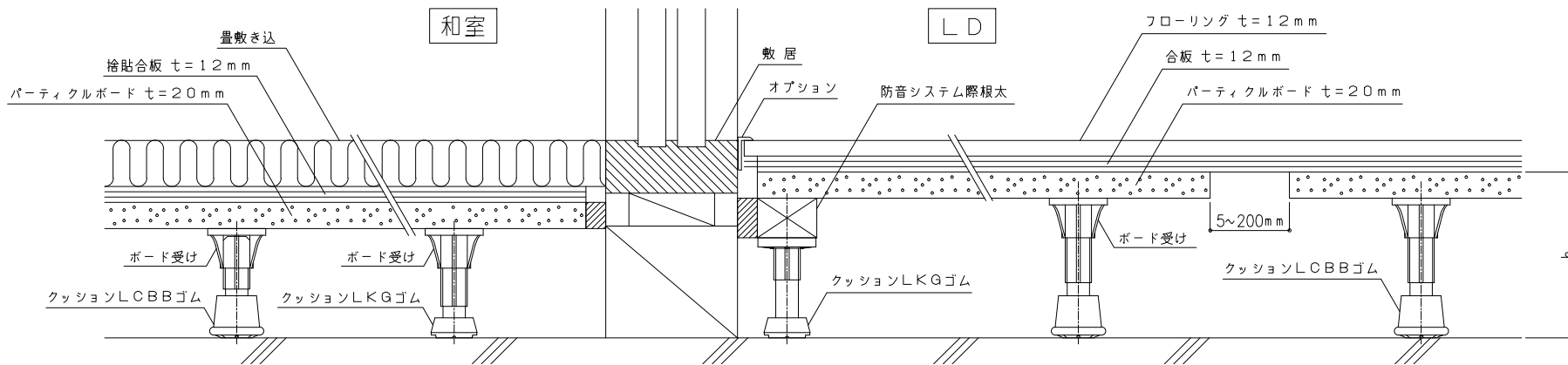
【ホームベース 760B：敷居廻り詳細図】
