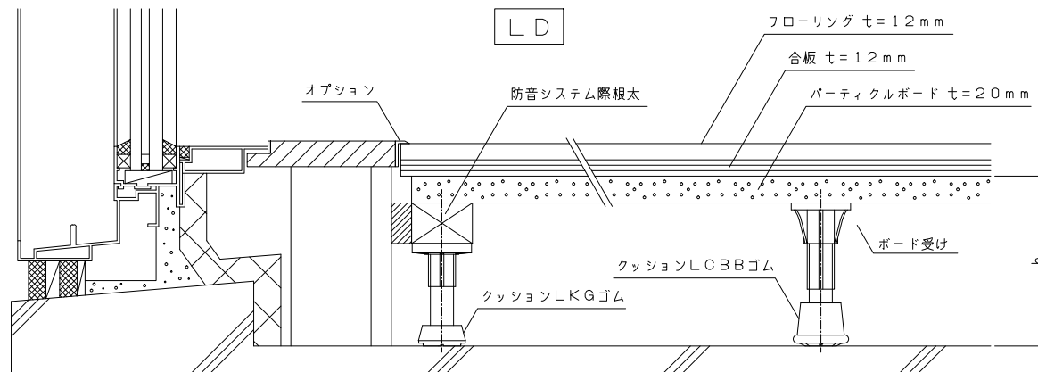
【ホームベース 760B：掃出し詳細図】
