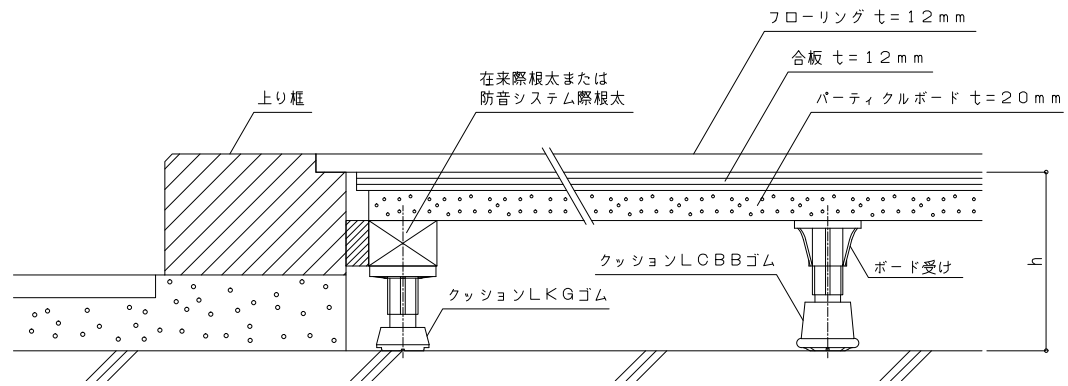
【ホームベース 760B：上り框取り合い図】
