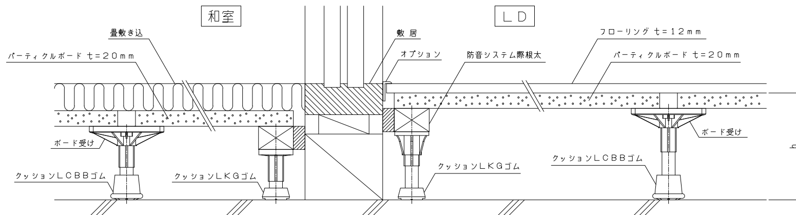
【ホームベース LCBB-N: 敷居廻り詳細図】
