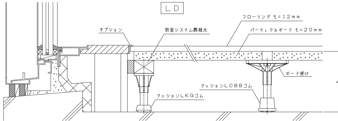
【ホームベース LCBB-N: 掃出し詳細図】
