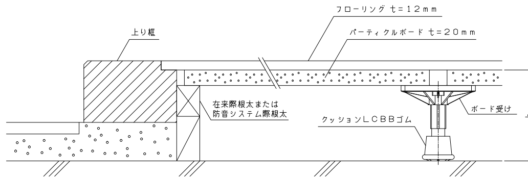
【ホームベース LCBB-N: 上り框取り合い図】
