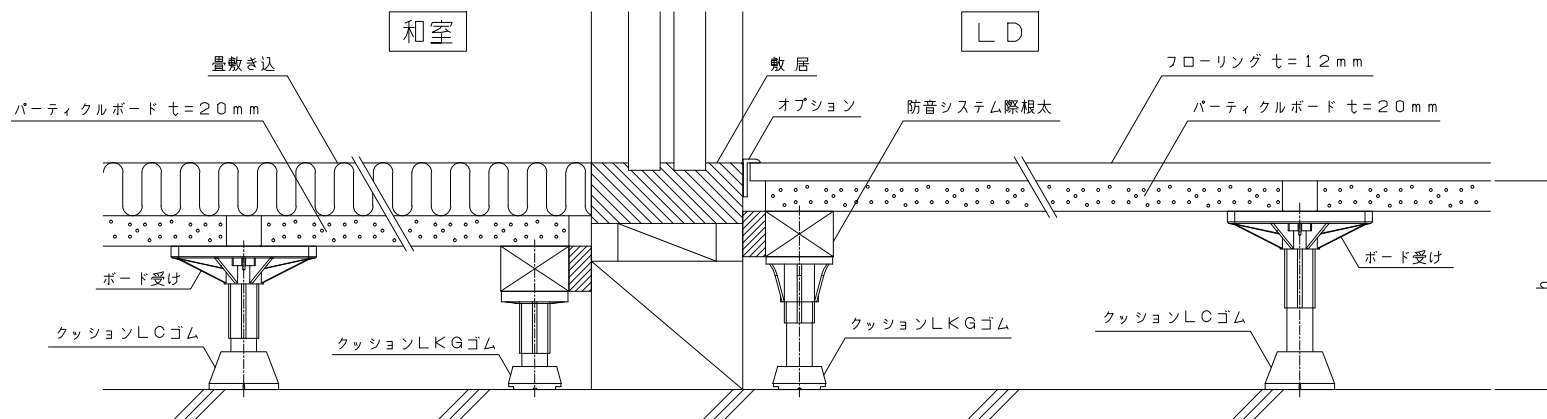
【ホームベース LC：敷居廻り詳細図】
