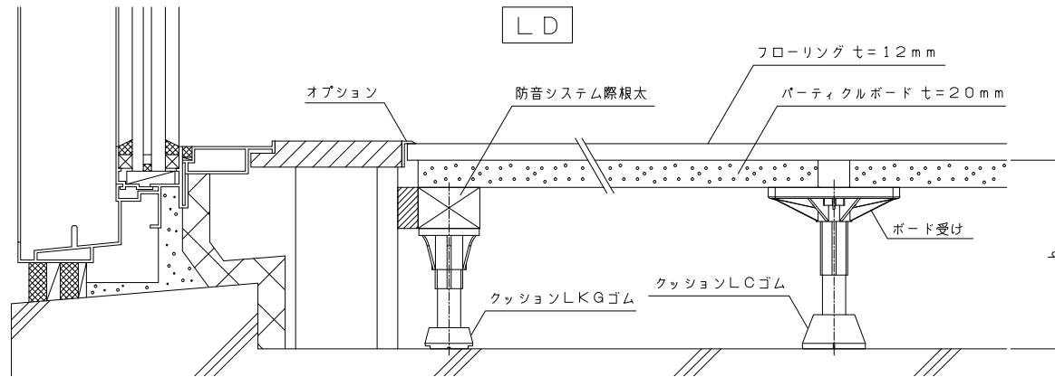
【ホームベース LC：掃出し詳細図】
