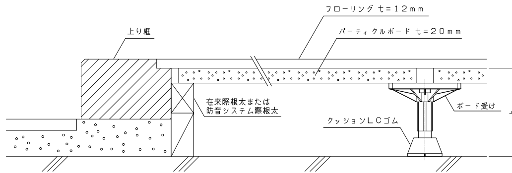
【ホームベース LC：上り框取り合い図】
