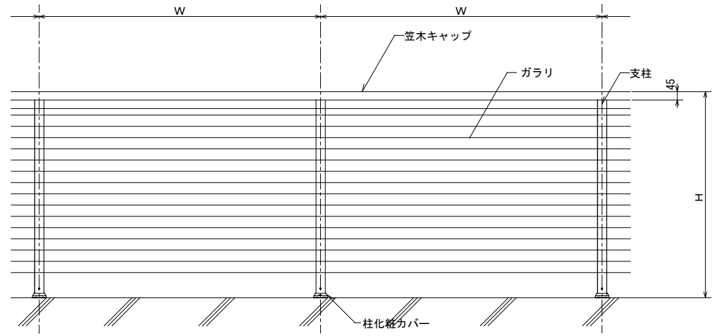
立面図
