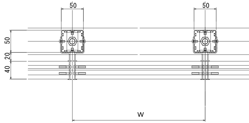
横断面図 S=1/3
