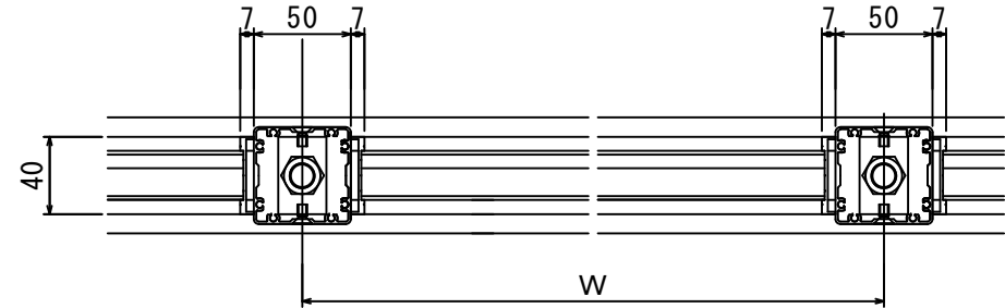
横断面図 S=1/3
