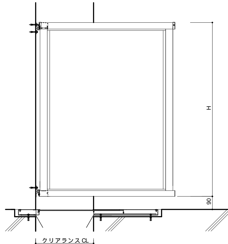
立面図
