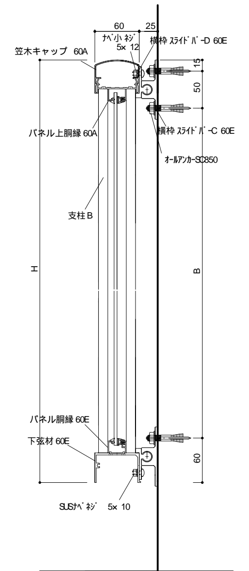
断面図
