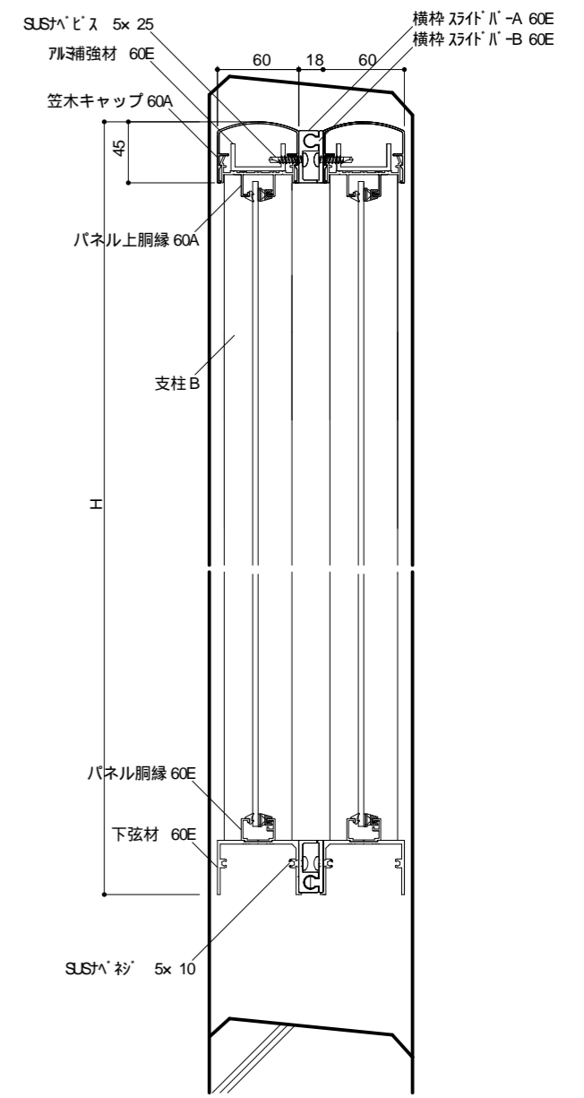
断面図 S=1: 5
