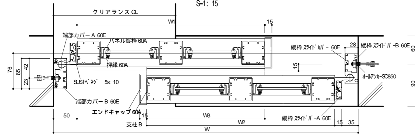
平面図 S=1: 5
