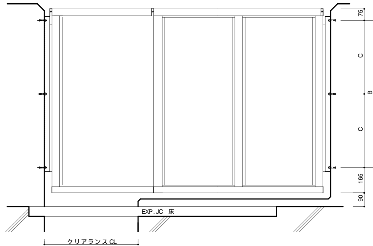
立面図 S=1: 15
