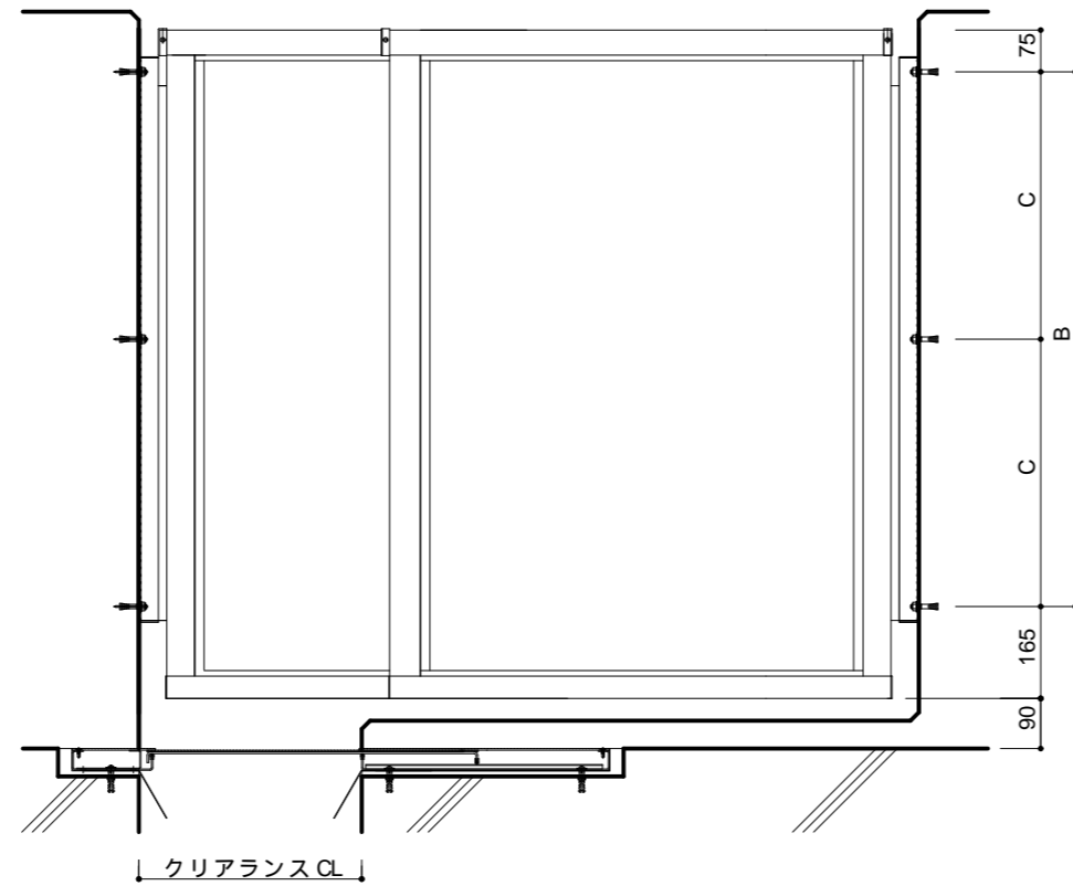
立面図
