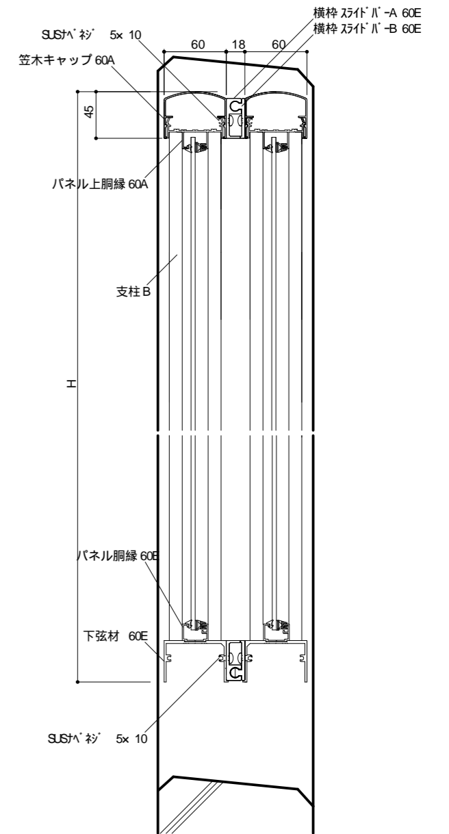
断面図
