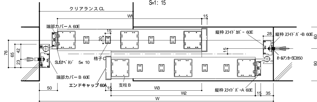
平面図
