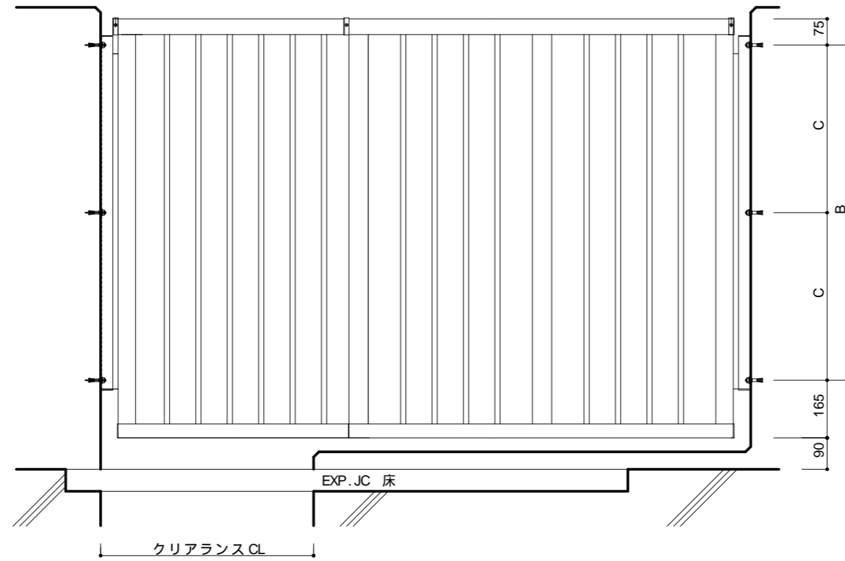
立面図
