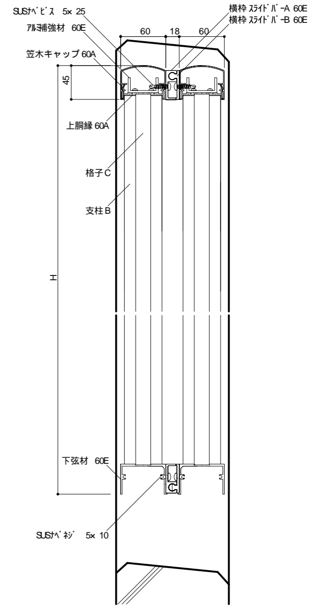
断面図
