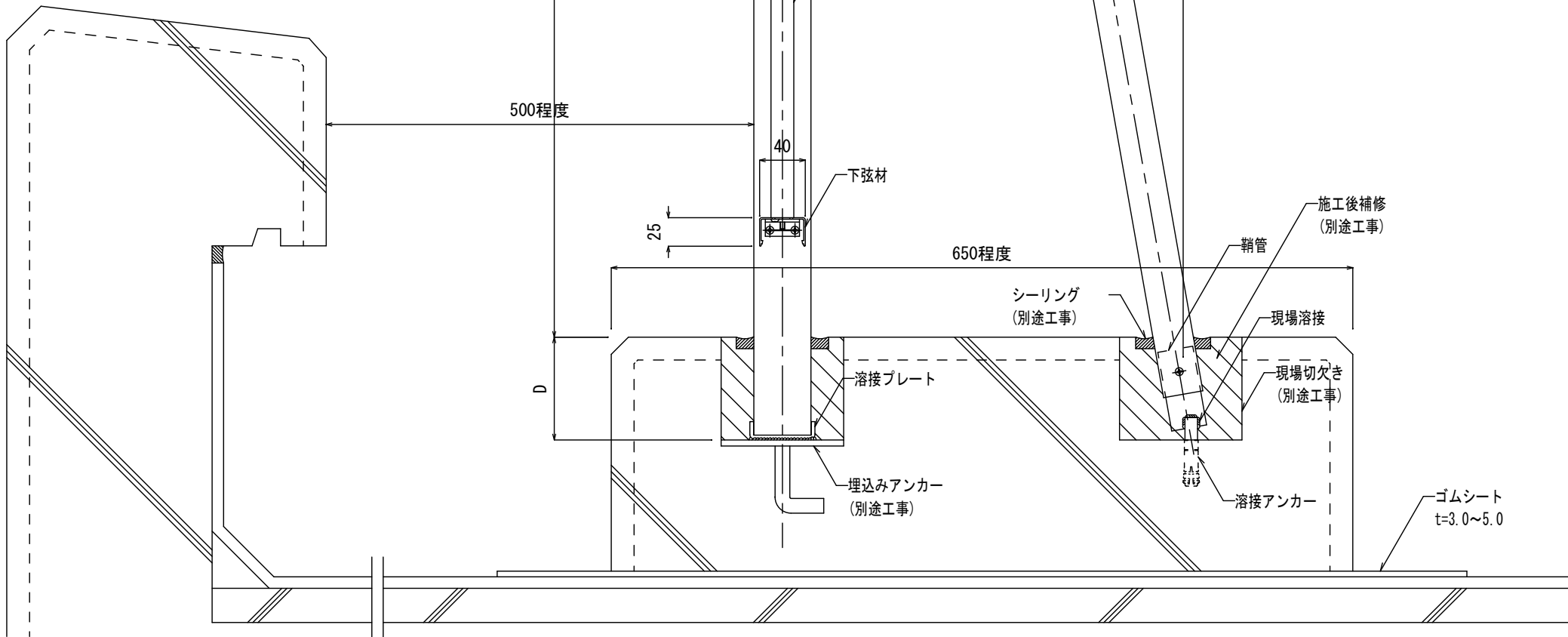
縦断面図 S=1/5
