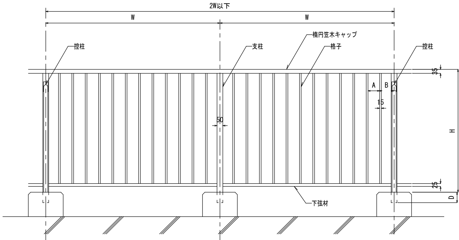
立面図 S=1/20
