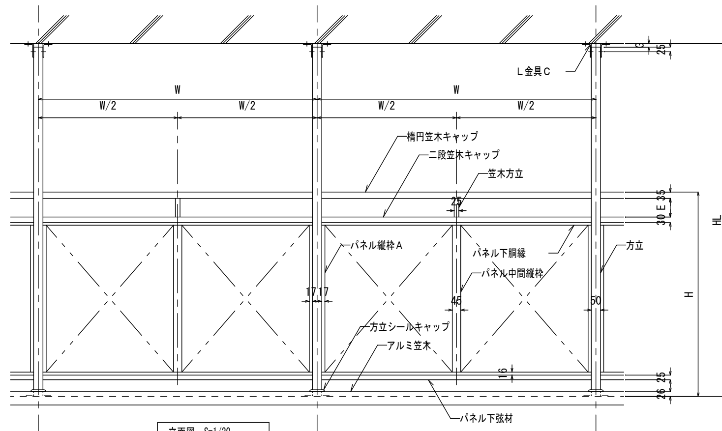
立面図 S=1/20
