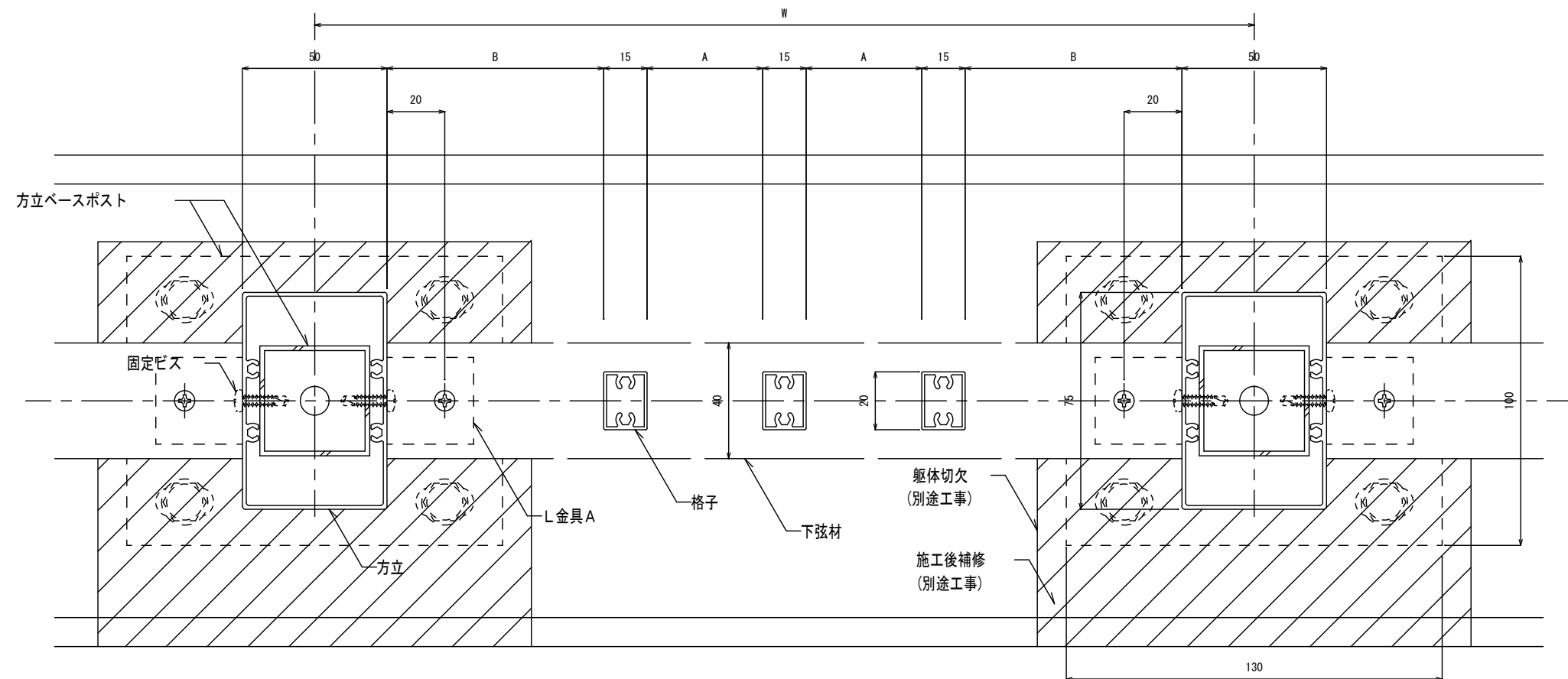
横断面図 S=1/2
